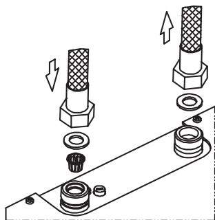
EPO.D - montage uniquement avec les tuyaux d'alimentation vers le haut
