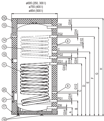
ABMESSUNGEN SW.INOX; SWZ.INOX
